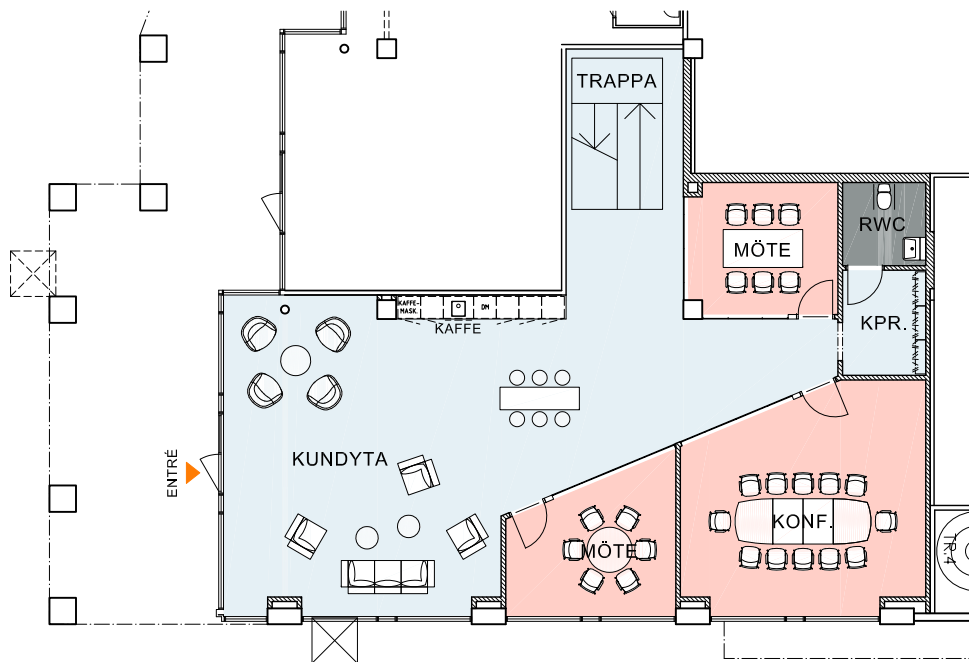
Plan bottenvåning
